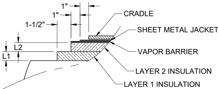
DOUBLE LAYER
