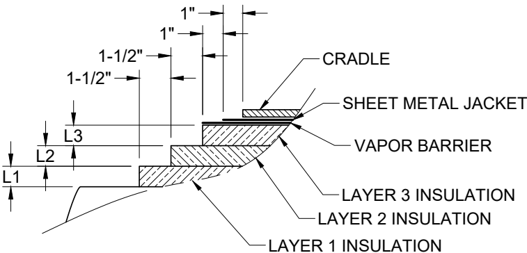
TRIPLE LAYER
