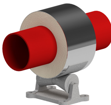
Calcium Silicate Roller (Medium Load)
