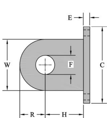
VIEW A-A
