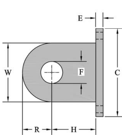
VIEW A-A
