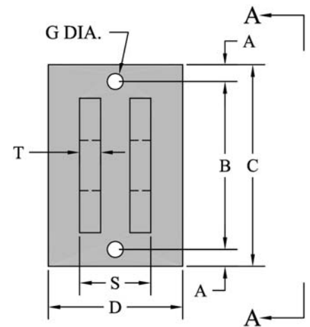
"C" TYPE LUG
